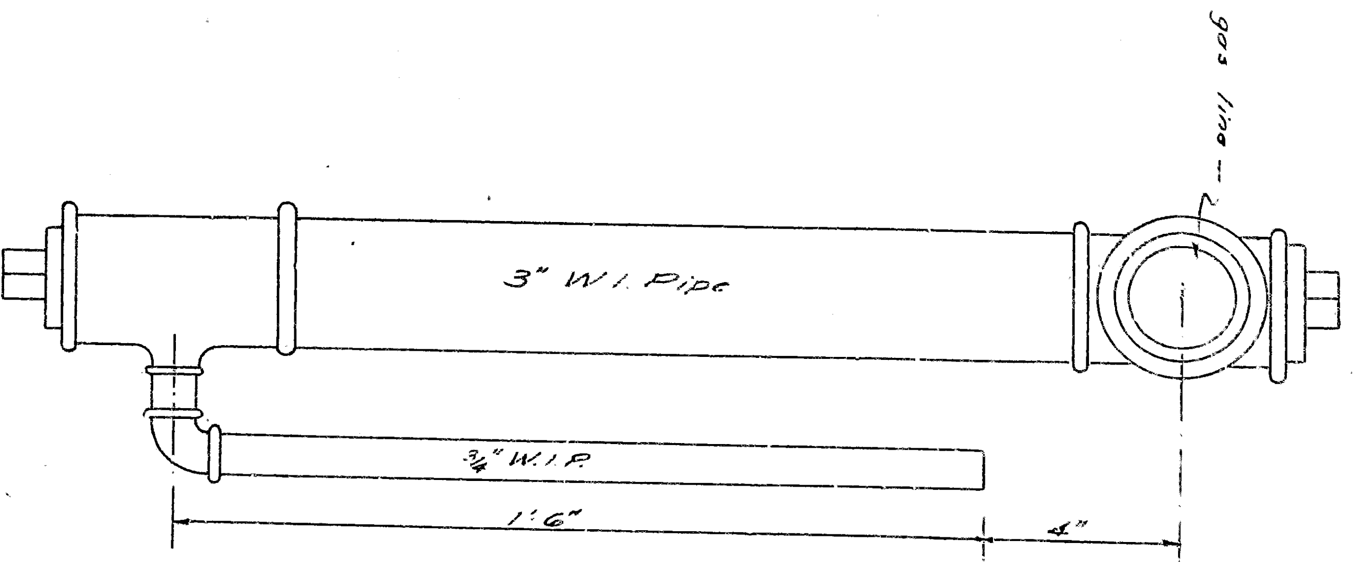
CONDENSATE TRAP
